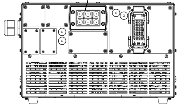
케이블 엔트리
