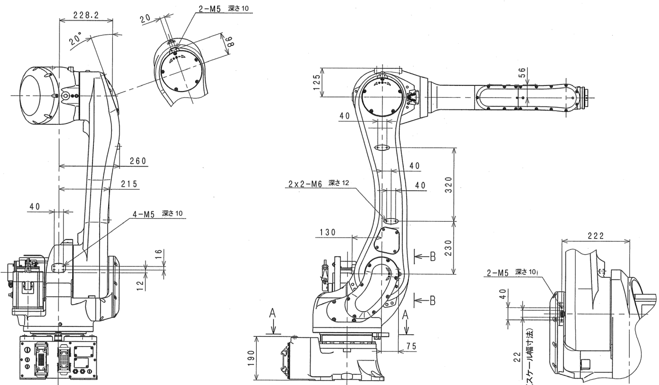
矢視 B-B
