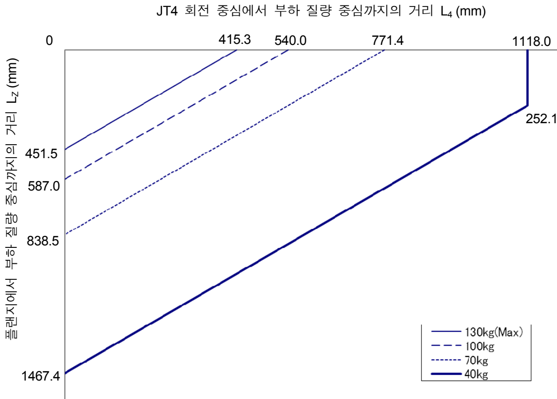
CP180L(고속 사양) 손목 부하 선도
