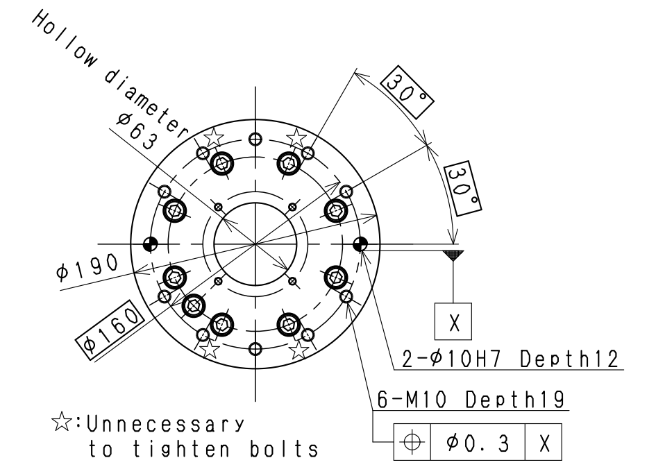
STANDARD FLANGE ※ Dimension:225
