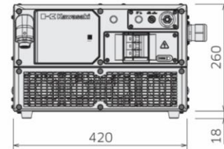
正面图
