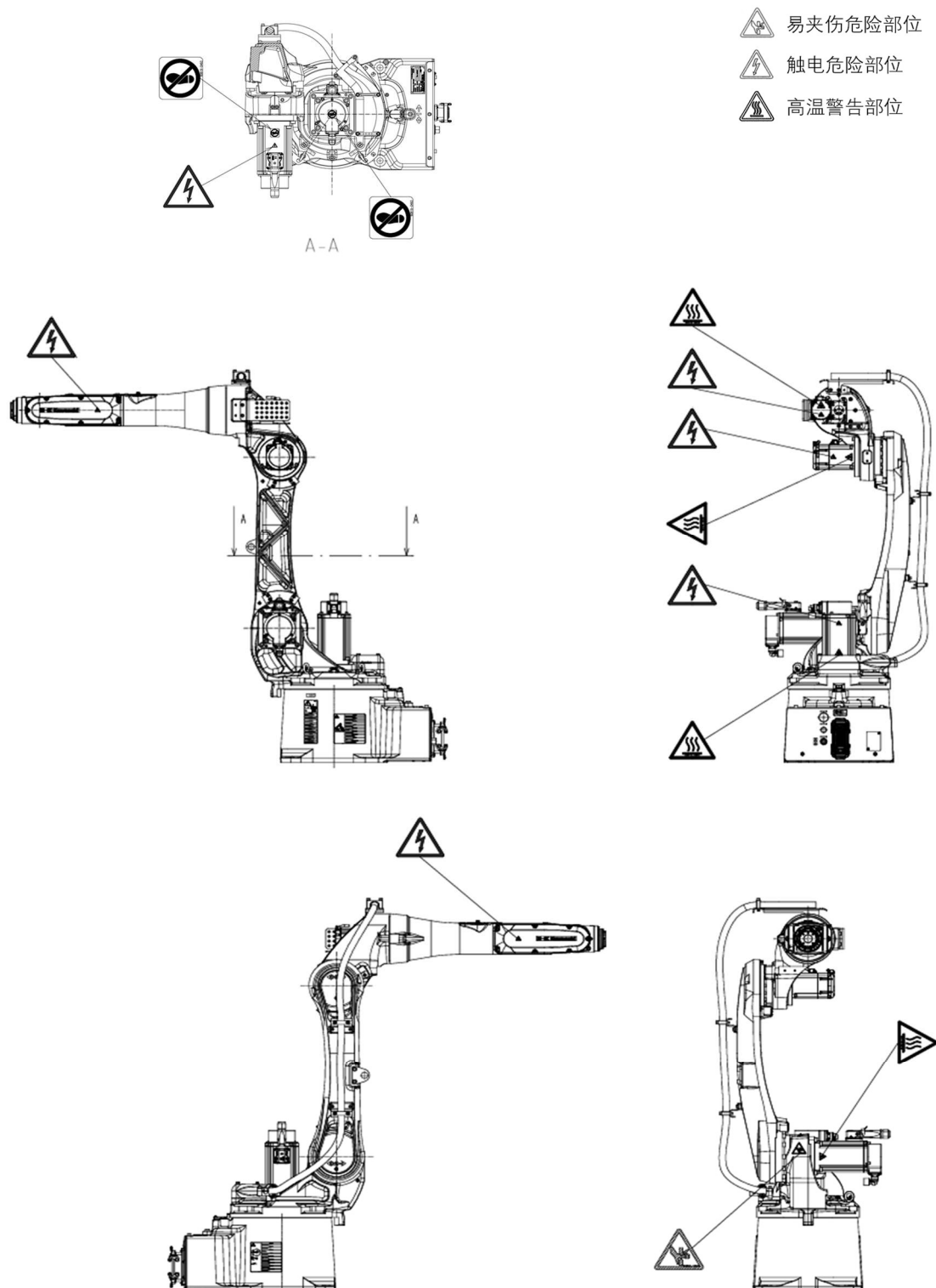
警告标签粘贴位置 (CF011N)
